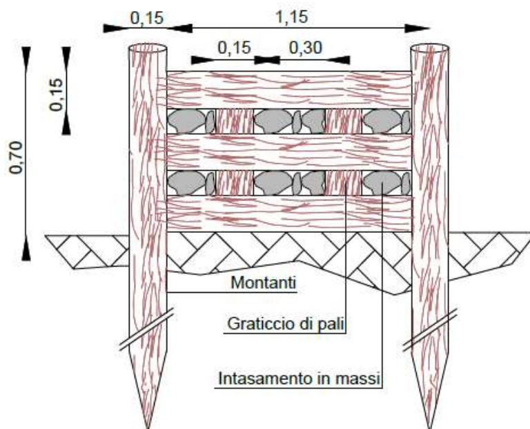
Figura 4: Tipologico palizzata in progetto.
